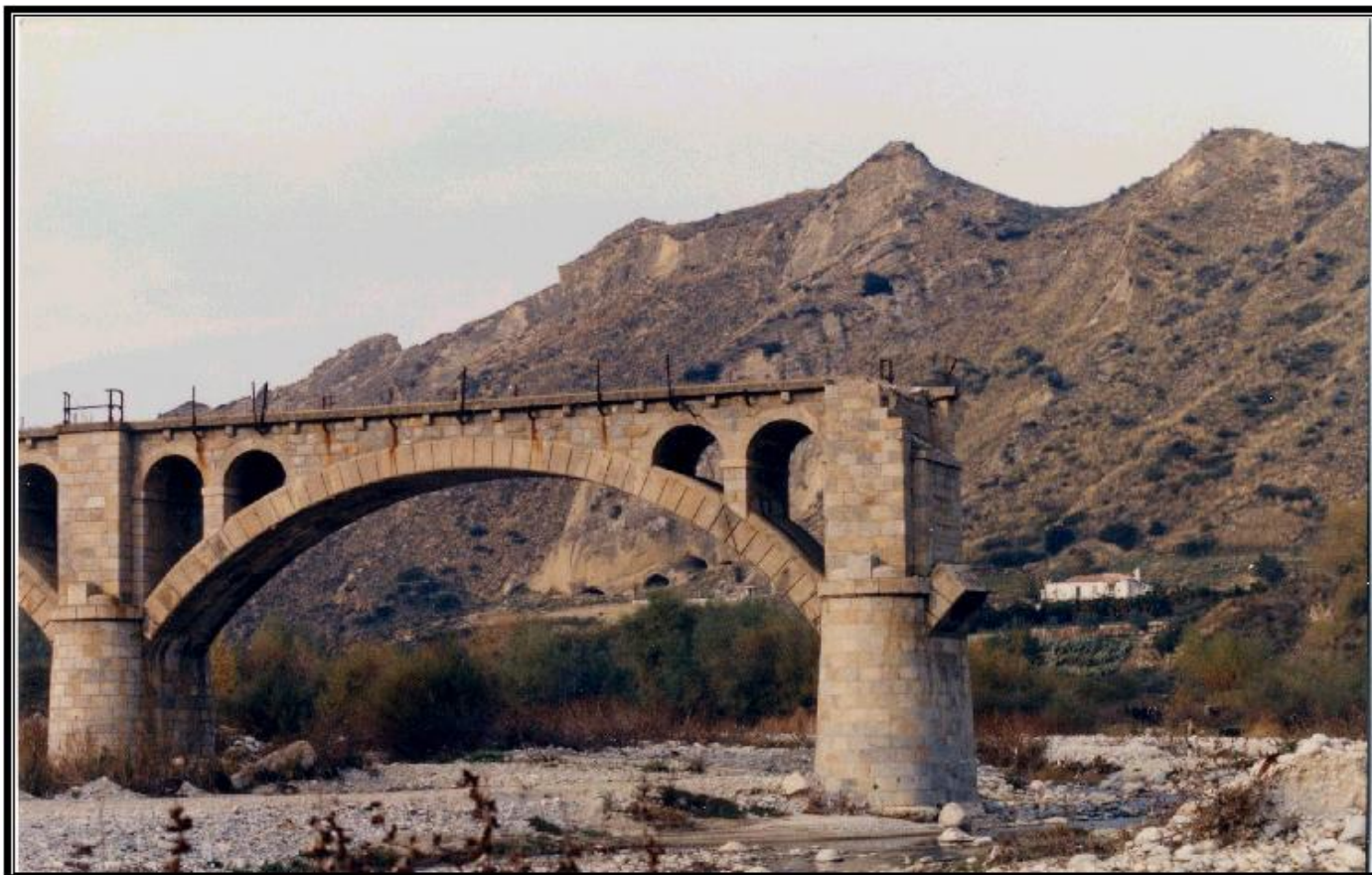
Ponte ferroviario crollato, fiume Tacina, alluvione del '73, Roccabernarda Niffi
